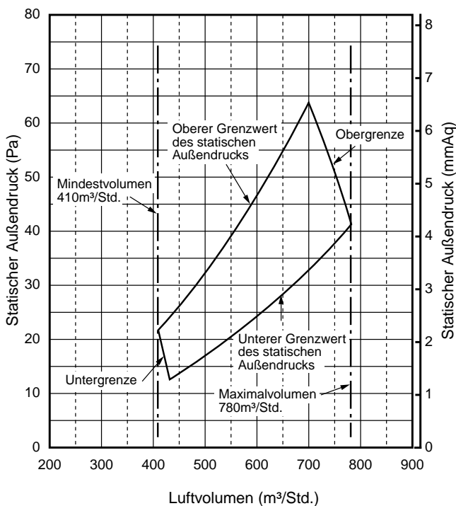
Abb. 2 RAS-M13GDCV-E, RAS-M13GDV-E
